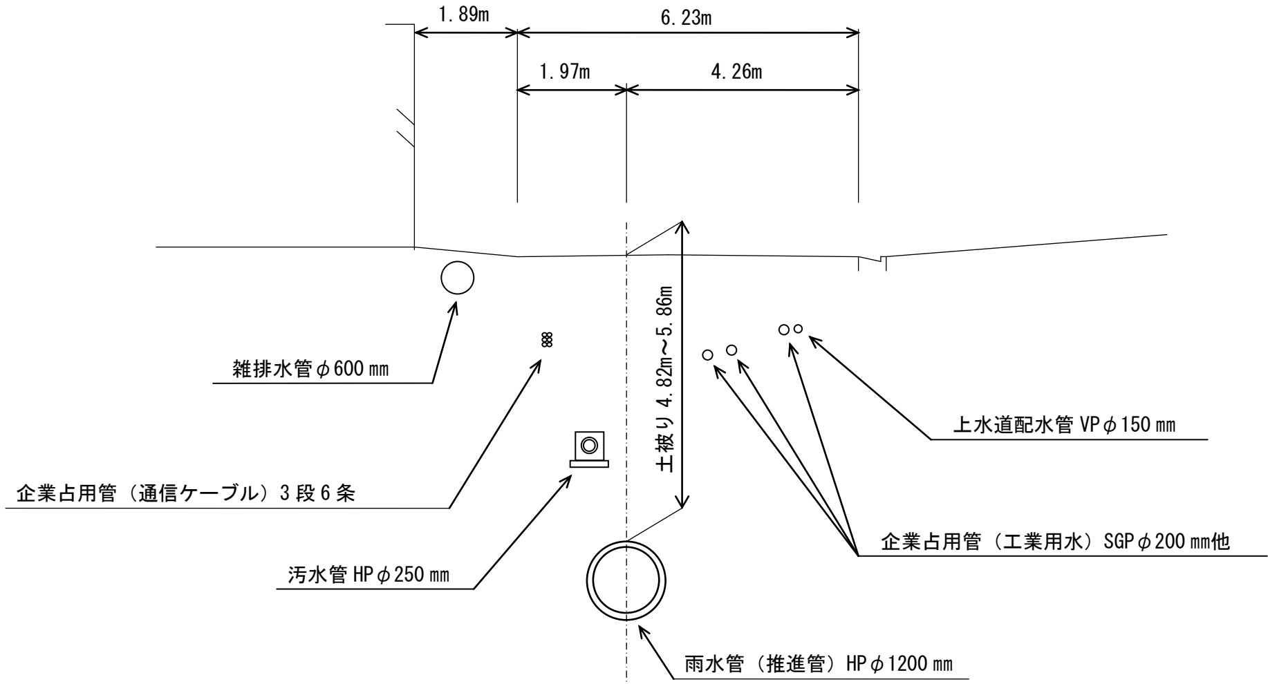
横断図
