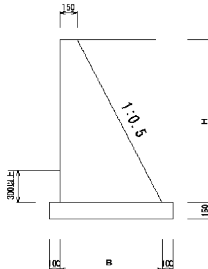
H ≤ 1500で輪荷重のある場合
