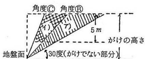
図-7 擁壁を要しないがけ又はがけの部分
