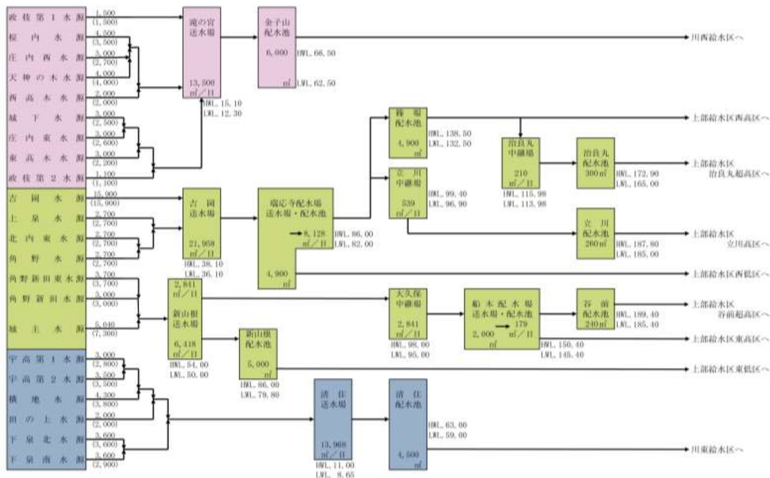
図 5 給水系統図
