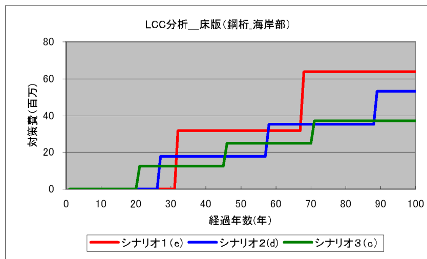
図 4-1 ライフサイクルコスト検討結果(例)
